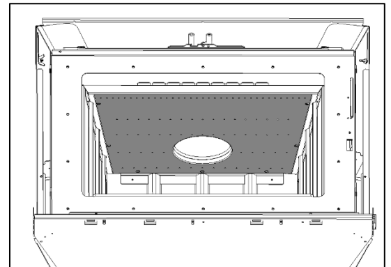
Illustration 2-2: Déflecteur de combustion secondaire à haute performance
