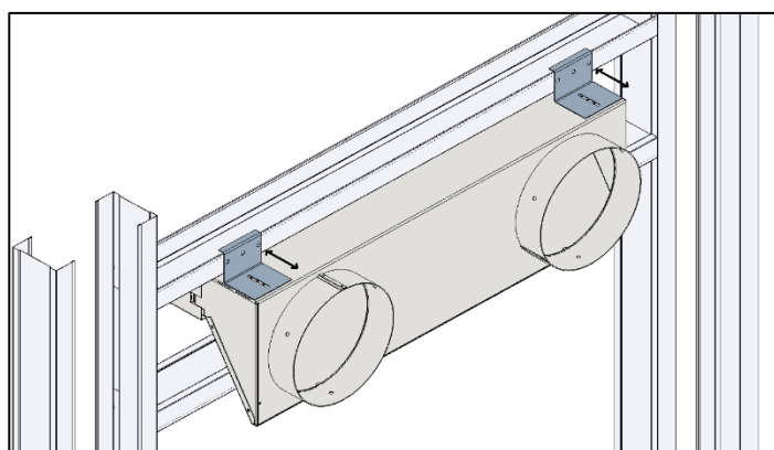
Illustration 3-25 : Supports ajustables de l'adaptateur linéaire conduit/grille
