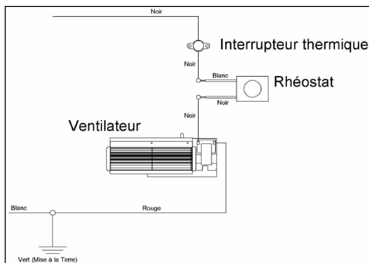
Illustration 3-43 : Diagramme électrique
