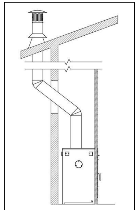
Illustration 3-6 : Installation extérieure
