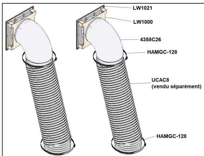
Illustration 3-21 : Schéma d'assemblage de l'ensemble KG540
