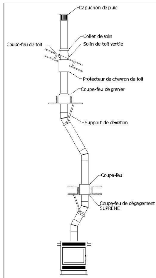
Illustration 3-7 : Installation avec déviation
