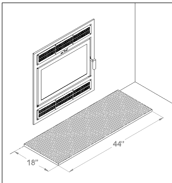
Figure 3-35 : Prolongement de l'âtre
