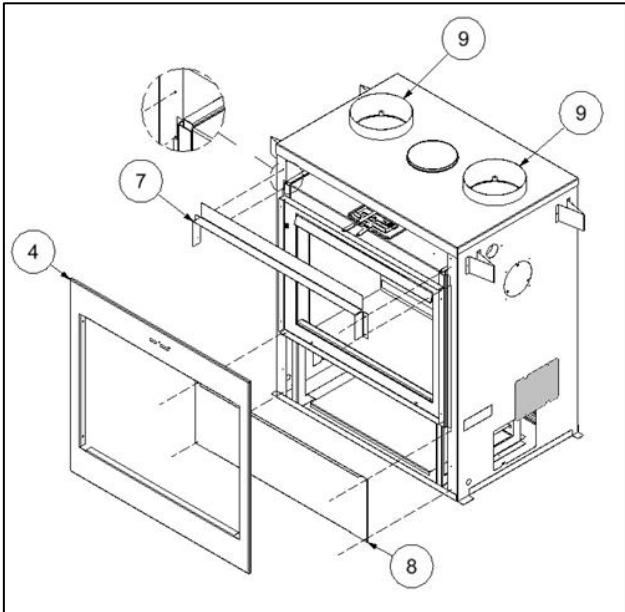
Illustration 3-16 : Installation de façade contemporaine
