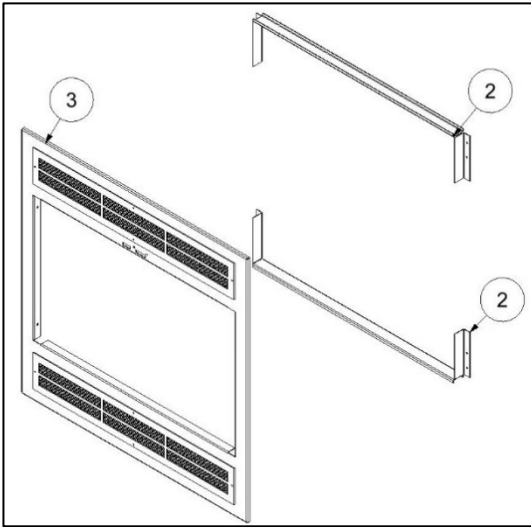
Illustration 3-14 : Composants de la façade traditionnelle rectangulaire
