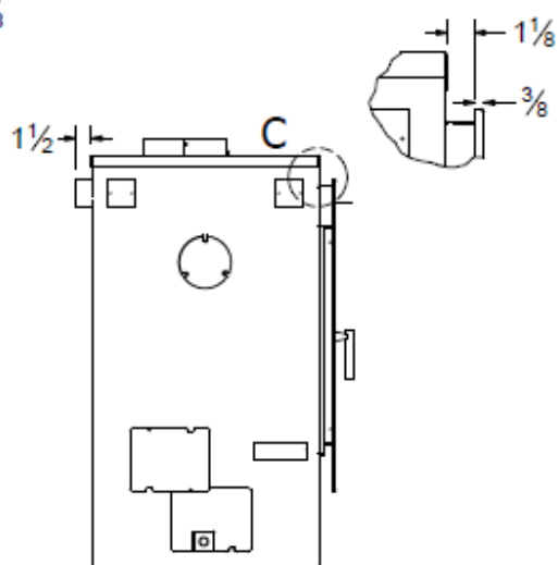
Illustration 2-3 : Dimensions Élégance 40 contemporain rectangulaire
