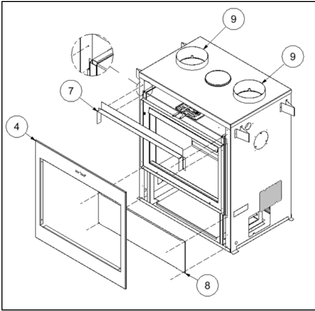
Illustration 3-17 : Installation de façade contemporaine
