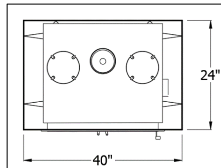
Illustration 3-1 : Installation mur droit
