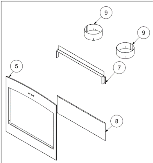
Illustration 3-19 : Composants de la façade contemporaine arquée
