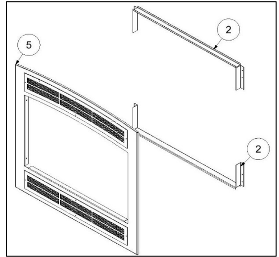
Illustration 3-15 : Composants de la façade traditionnelle arquée
