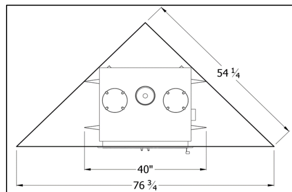
Illustration 3-2 : Installation en coin
