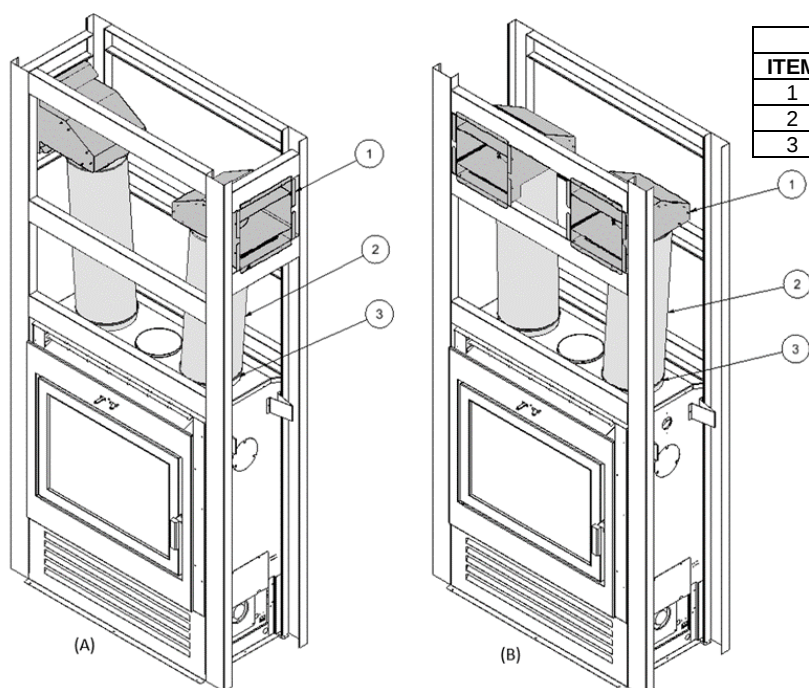
Illustration 3-10: Éléance ST 8'' conduit par gravité à grilles doubles avec sorties d'air chaud (A) latérales et (B) frontale ou dorsale
